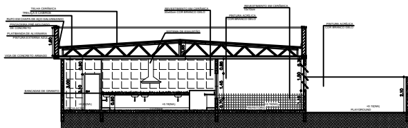
CORTE A-A Escola 1/100
