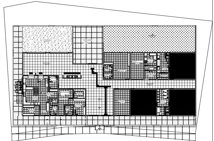
PAGINAÇÃO DE PISOS Escola 1/125
