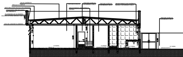
CORTE B-B Escola 1/100
