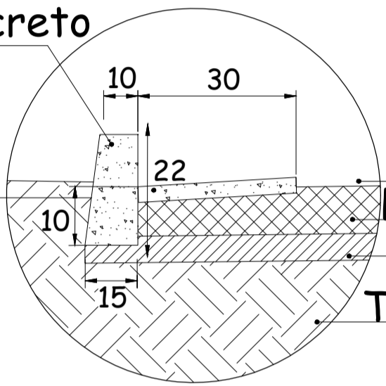
DETALHE 01 SEM ESCALA
