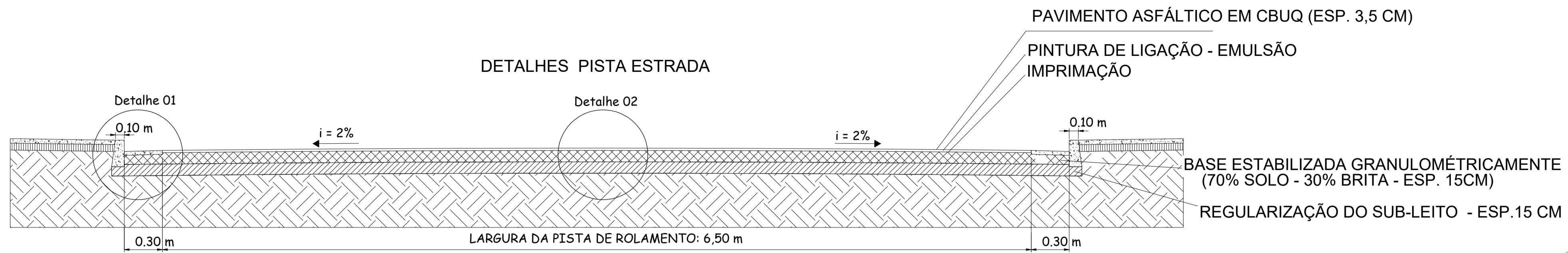
CORTE - PISTA SEM ESCALA
