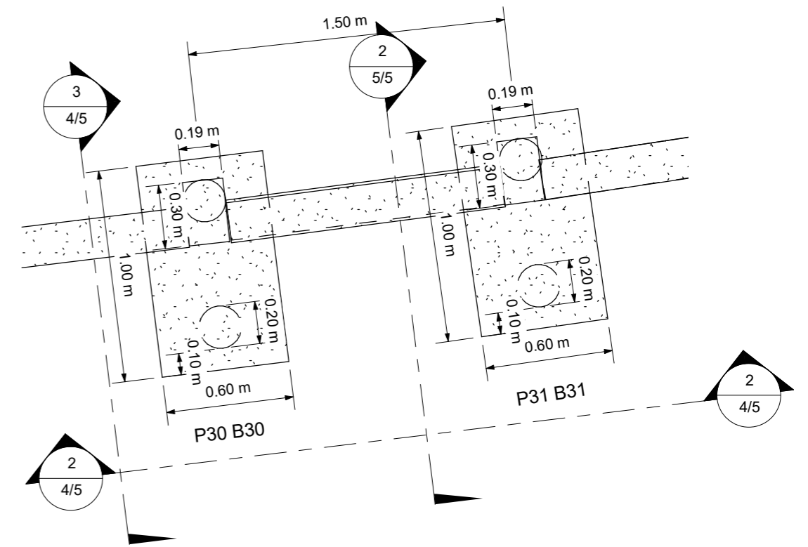
4 Detalhe da fundação 1 : 25
