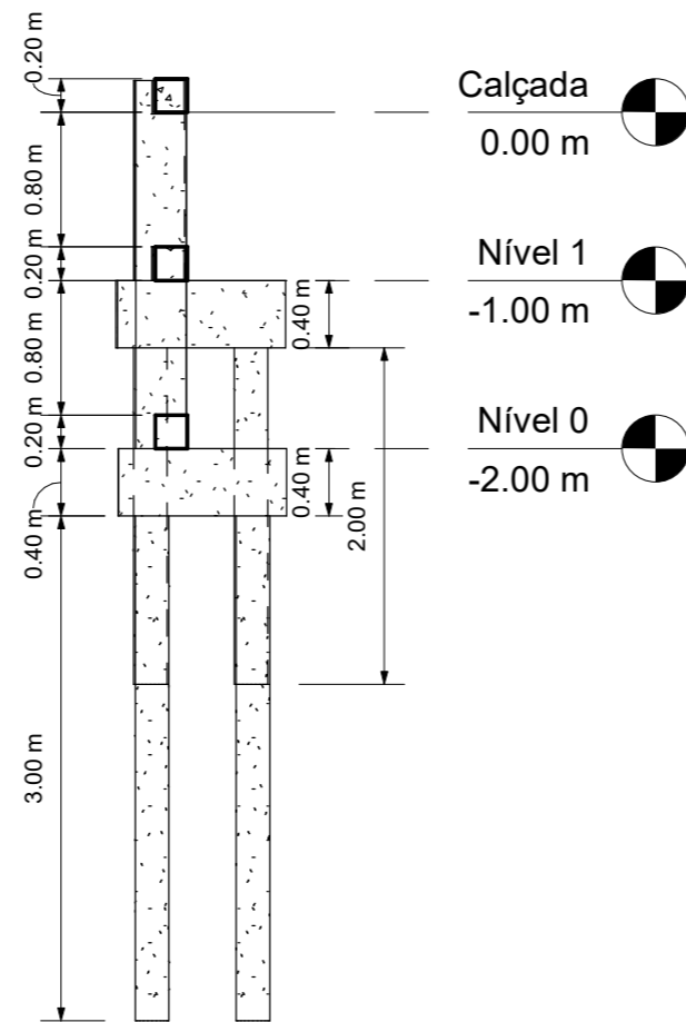
3 Corte BB 1 : 50
