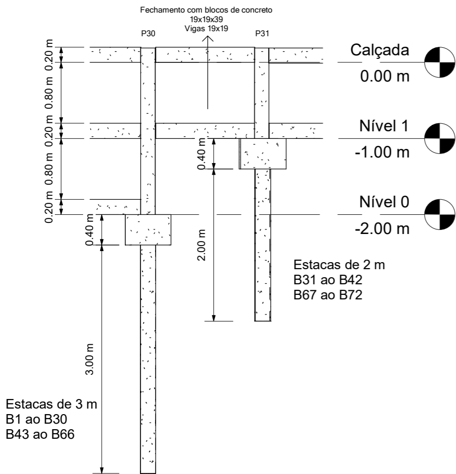
2 Corte AA 1 : 50
