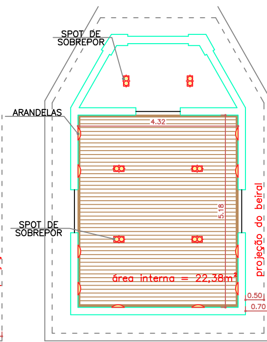
PLANTA FORRO E ILUMINAÇÃO ESC. 1:100
