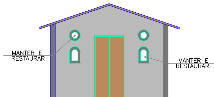
VISTA FRONTAL (após frontão de entrada) ESC. 1:75
