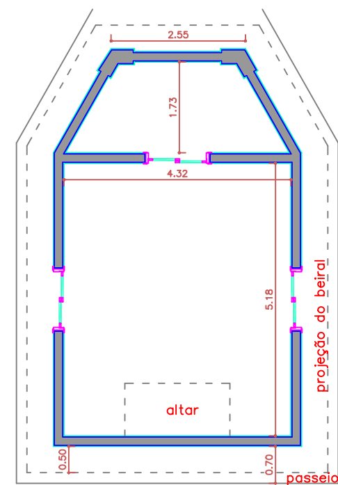
PLANTA BAIXA ESC. 1:100
