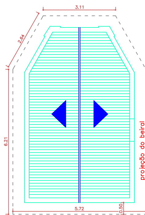
PLANTA COBERTURA ESC. 1:100
