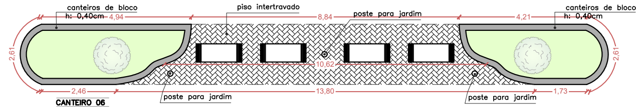
CANTEIRO 06 ESC. 1:125
