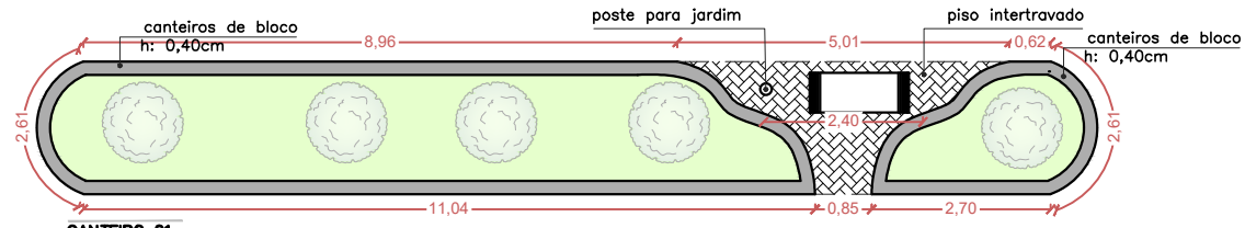
CANTEIRO 01 ESC. 1:125
