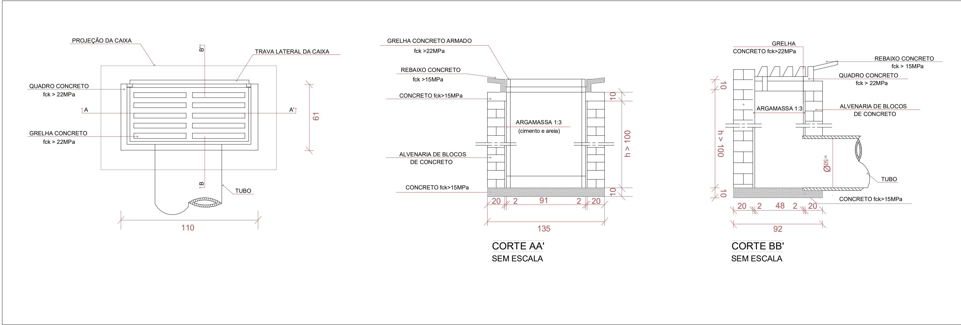
DETALHE 1 - BOCA DE LOBO SÓ DE SAÍDA (Á CARGO DA PREFEITURA) Sem escala
