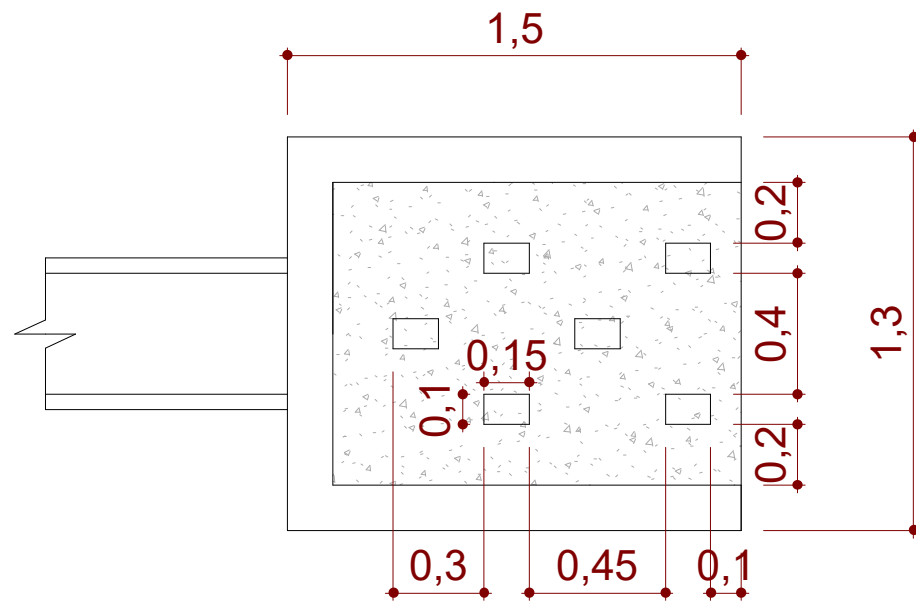
4 Detalhe do dissipador ESCALA - 1 : 25
