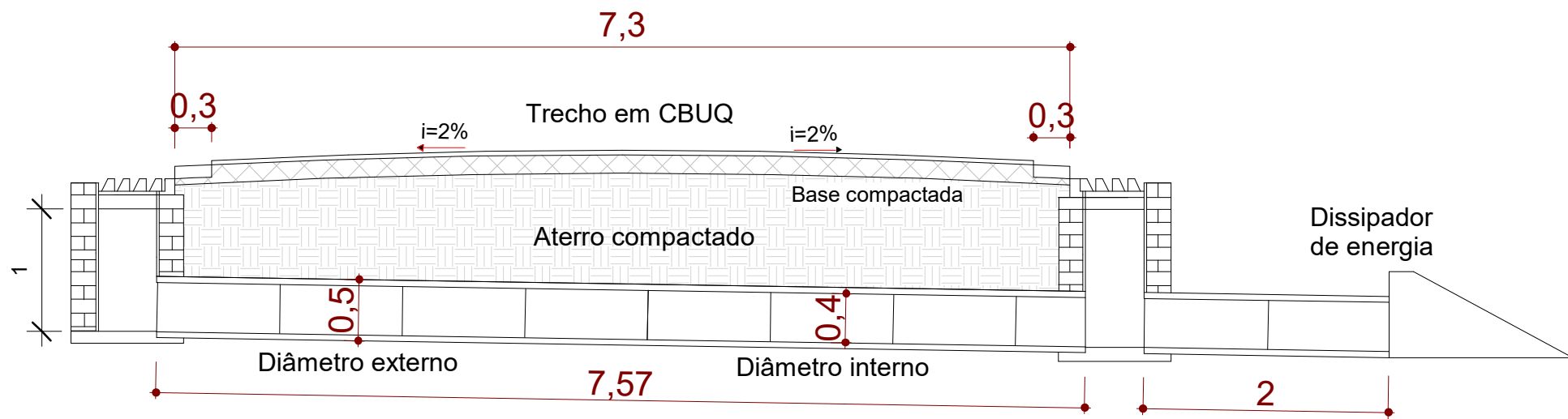
DETALHE 1 - DRENAGEM, BOCA DE LOBO, BUEIRO (Á CARGO DA PREFEITURA) Escala 1:50
