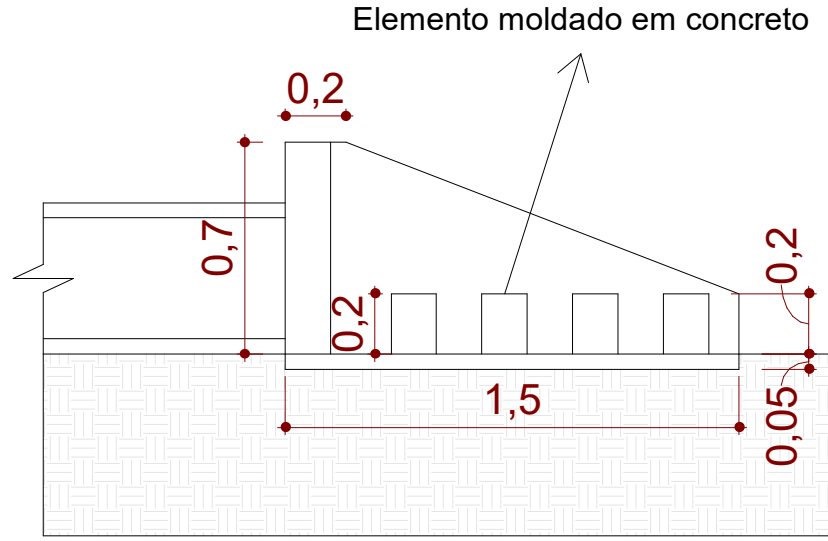
CORTE 01 SEM ESCALA
