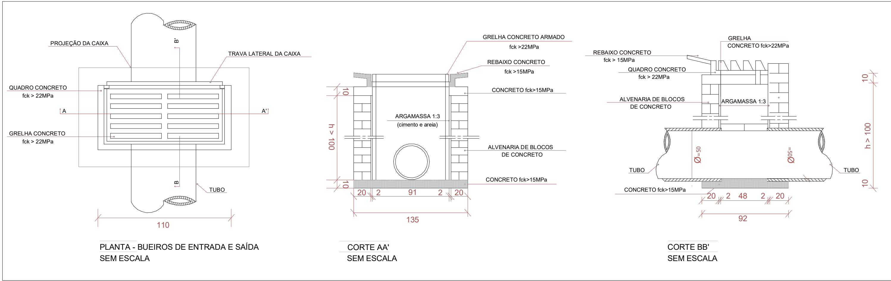
DETALHE 2 - BOCA DE LOBO ENTRADA E SAÍDA (Á CARGO DA PREFEITURA) Sem escala
