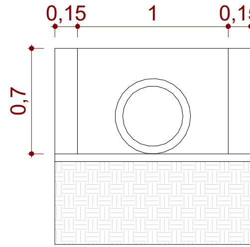
CORTE 02 SEM ESCALA
