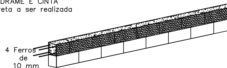
CINTA DE AMARRAÇÃO muros a serem ampliados
