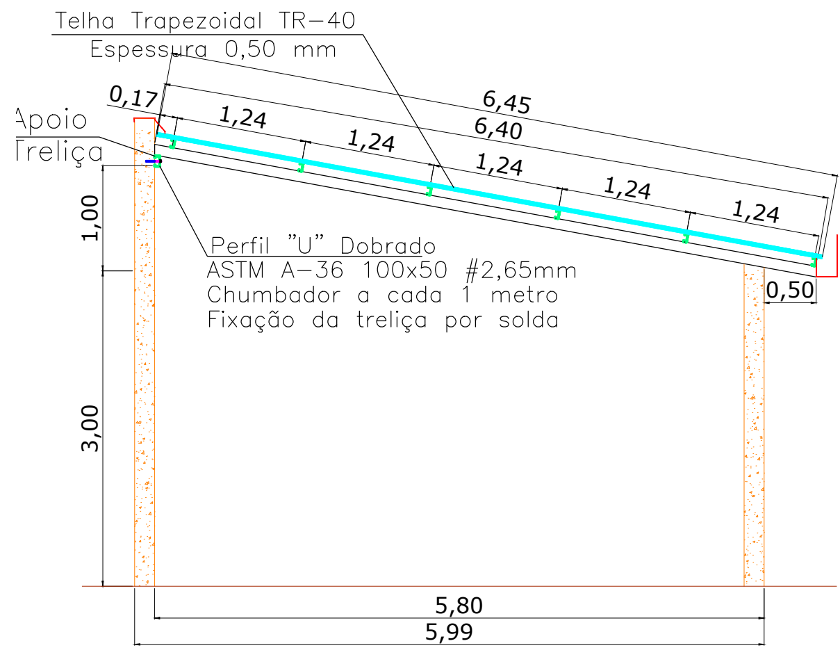
Vista Lateral -ESCALA: 1:50
