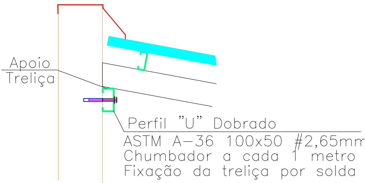
Detalhe Apoio Treliza
